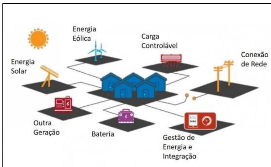
Figura 1 – Representação Microrrede
