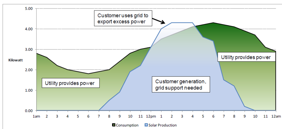
Gráfico 2.1. Curvas típicas de produção e consumo de um pequeno consumidor detentor de um sistema fotovoltaico
