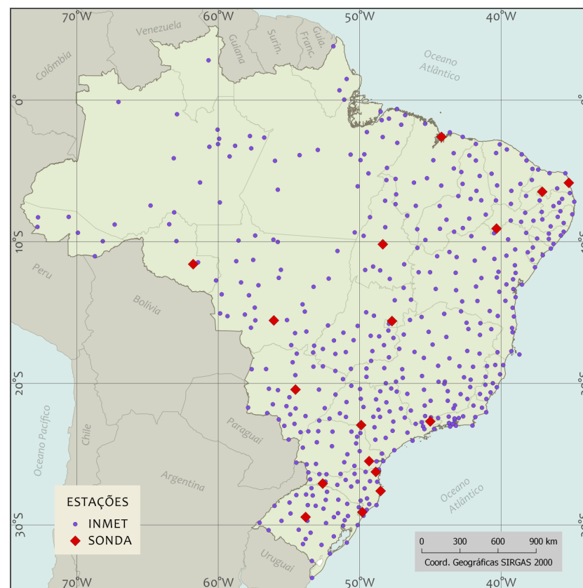
Figura 29. Localização das estações da rede SONDA e das EMA's da rede de observação meteorológica operada pelo INMET utilizadas na validação do Atlas (adaptado de: http://www.inmet.gov.br/portal/index.php?r=estacoes/estacoesAutomaticas ).
