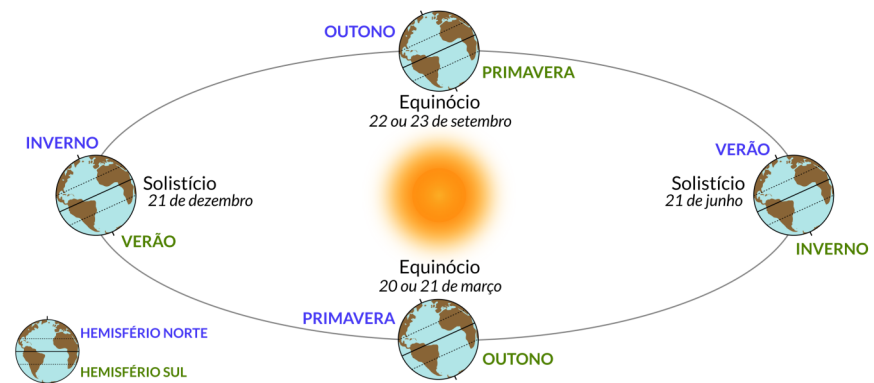
Figura 8. A geometria Sol-Terra determina as estações do ano e a duração do dia. O Sol está posicionado sobre a linha dos Tropicó de Câncer e de Capricórnio nos dias de solstício e posicionado sobre o Equador nos equinócios.
