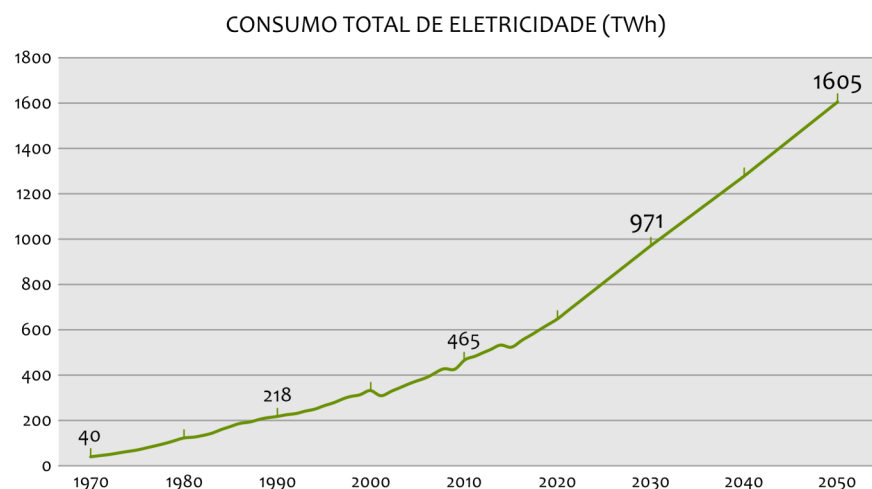
Figura 5. Série Histórica do Consumo Total de Energia Elétrica no Brasil (1970-2015) e previsão de demanda para o período 2020-2050. Fonte: Adaptado de MME (2017), MME (2016b).
